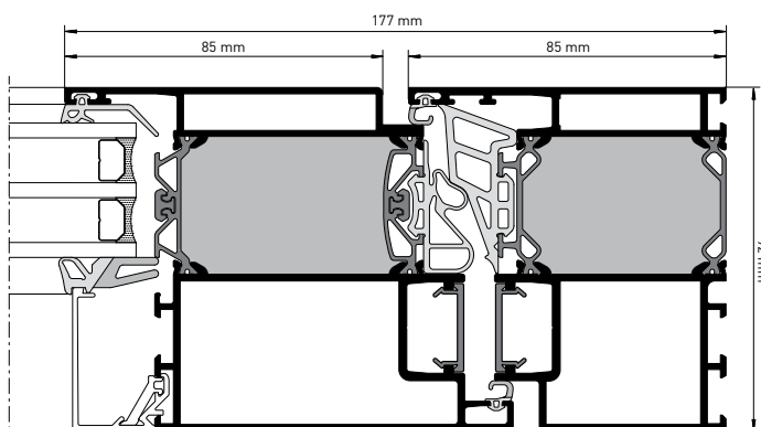
Dveřní systém D 92 UD, boční řez
